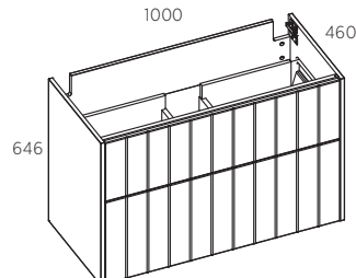
PRAUSTUVO SPINTELĖ 100 (2 dalių)
