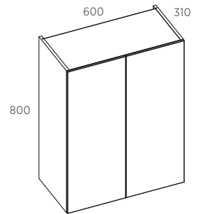
ŠONINĖ SPINELĖ 600x800x310
