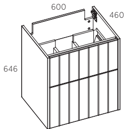
PRAUSTUVO SPINTELĖ 60 (2 dalių)
