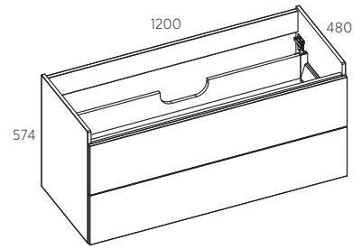
PRAUSTUVO SPINTELĖ 120 NSS
