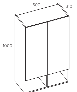
ŠONINĖ SPINELĖ 600x1000x310
