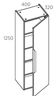
AUKŠTA ŠONINĖ SPINTELĖ (maža)
