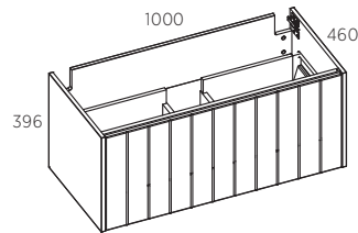
PRAUSTUVO SPINTELĖ 100 (2 dalių)
