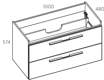
PRAUSTUVAI SU STALVIRŠIU 100
