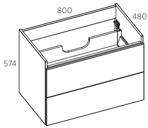
PRAUSTUVO SPINTELĖ 80 NSS
