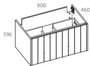
PRAUSTUVO SPINTELĖ 80 (2 dalių)
