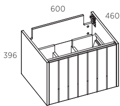
PRAUSTUVO SPINTELĖ 60 (2 dalių)
