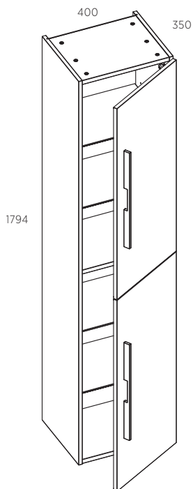
AUKŠTA ŠONINĖ SPINTELĖ NSS
