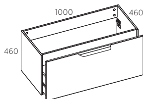
PRAUSTUVO SPINTELĖ 100 (2 stalčiai)
