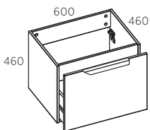
PRAUSTUVO SPINTELĖ 60 (2 stalčiai)
