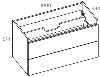
PRAUSTUVO SPINTELĖ 100 NSS
