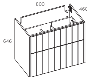
PRAUSTUVO SPINTELĖ 80 (2 dalių)
